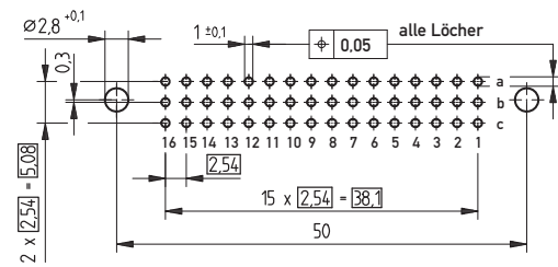
Leiterplatten-Lochbild
