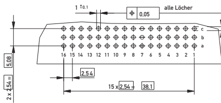
Leiterplatten-Lochbild
