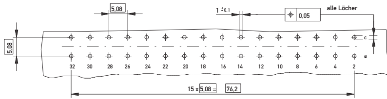
Leiterplatten-Lochbild
