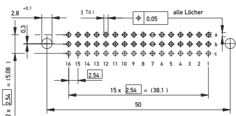
Leiterplatten-Lochbild
