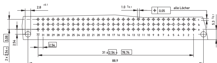
Leiterplatten-Lochbild
