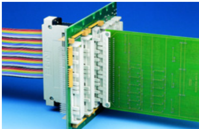
Codierleiste UE montiert auf einer Rückwandplatine mit Peripherieschnittstelle
