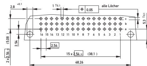
Leiterplatten-Lochbild
