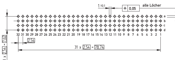
Leiterplatten-Lochbild
