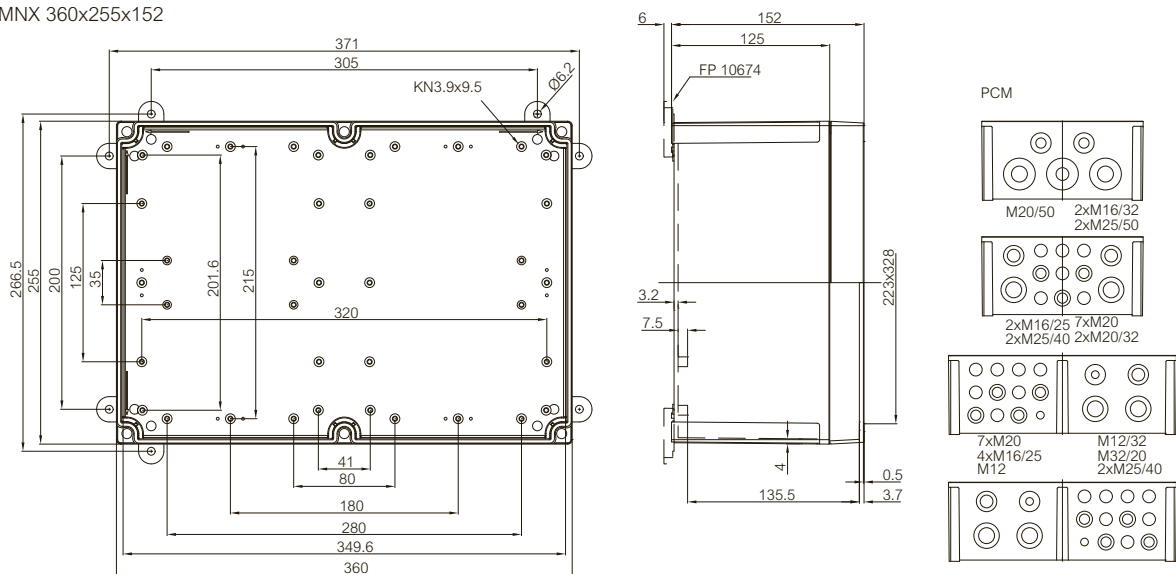
MNX 360x255x152
