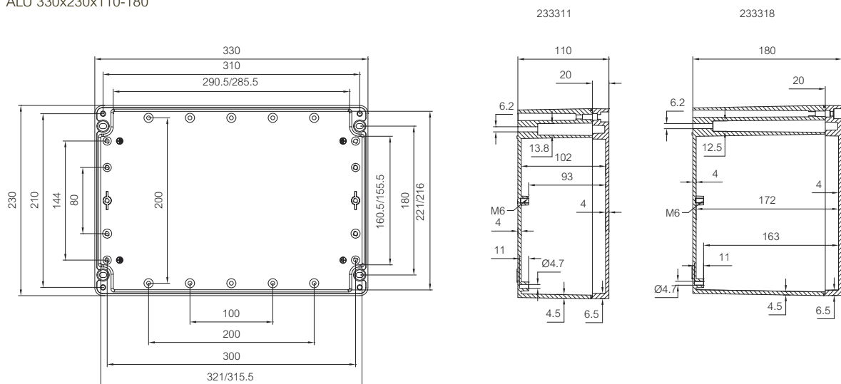
ALU 330x230x110-180
